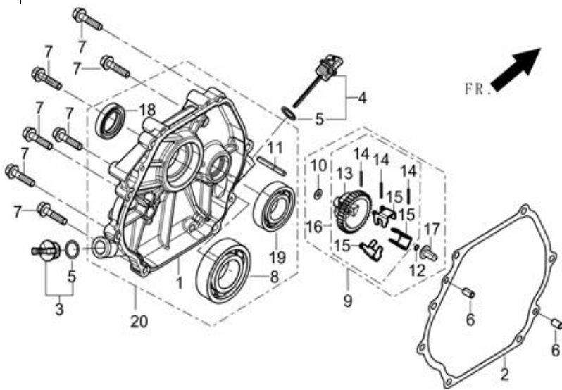
图 3 : 曲轴箱盖部件 + 调速齿轮部件(E01)
