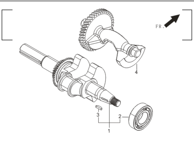
图 4 : 曲柄连杆组件(E03)
