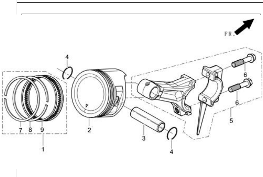
图 5 : 油环组合/曲柄连杆组件 (E03)
