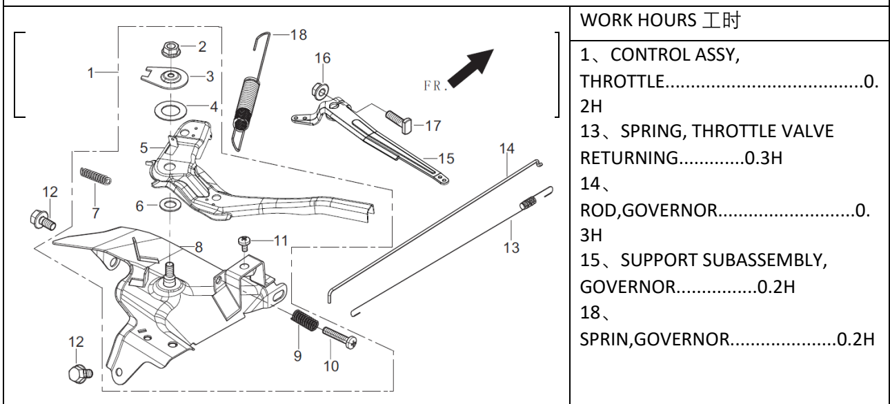
图 14 : 油门操纵部件 (E13)
